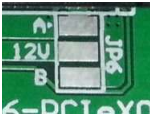
図 8: JP6 によるホスト側/デバイス側 PCIe の 12V 電源供給
