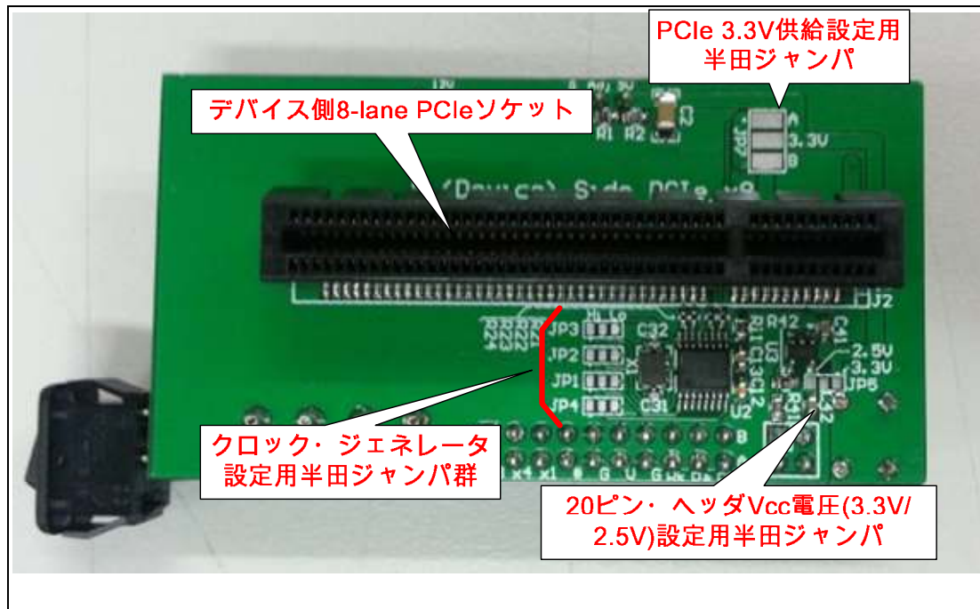
図 2: アダプタ基板のデバイス接続側
