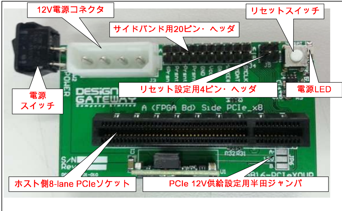
図 1: アダプタ基板のホスト接続側
