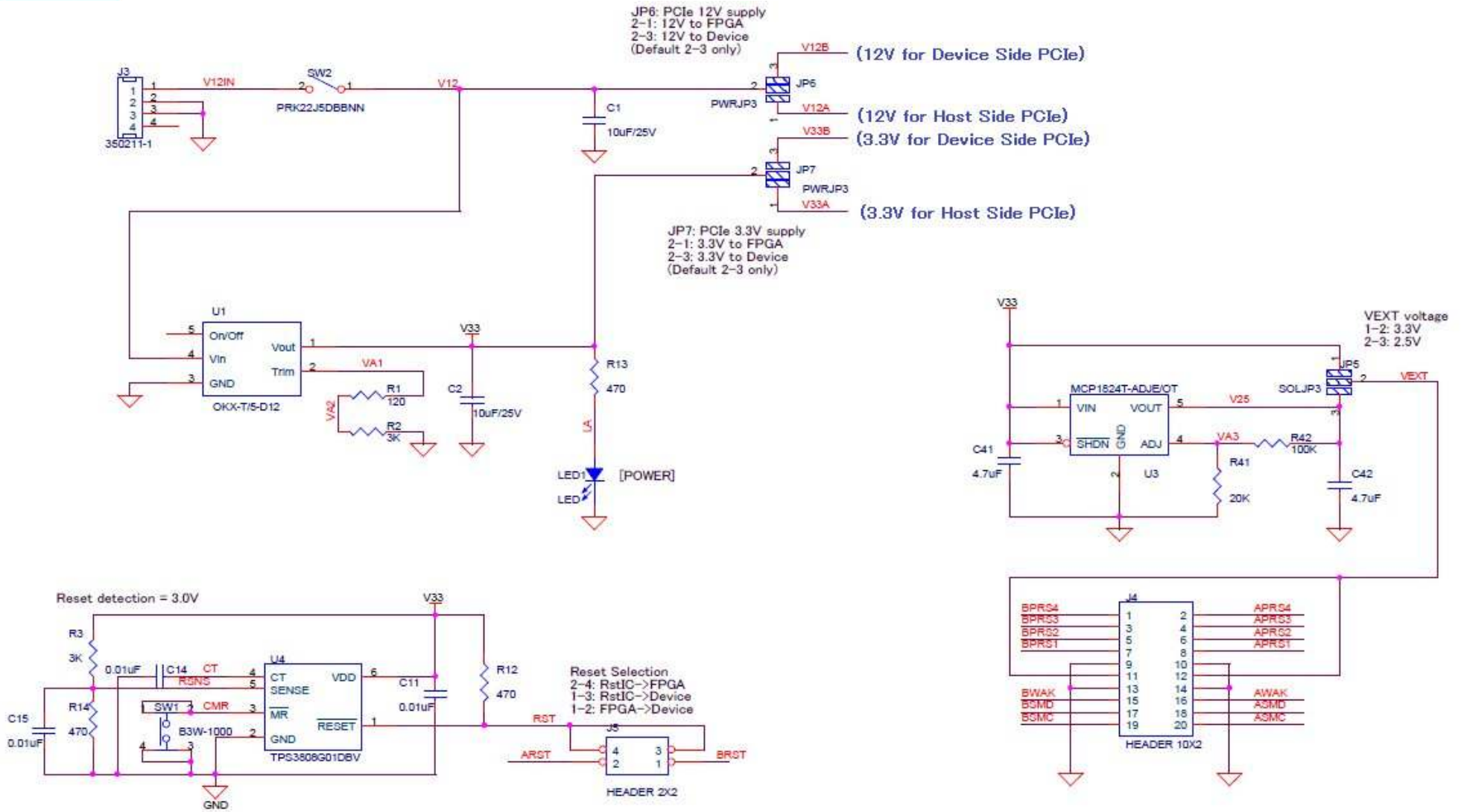
図 11: アダプタ回路図 (1/2)
