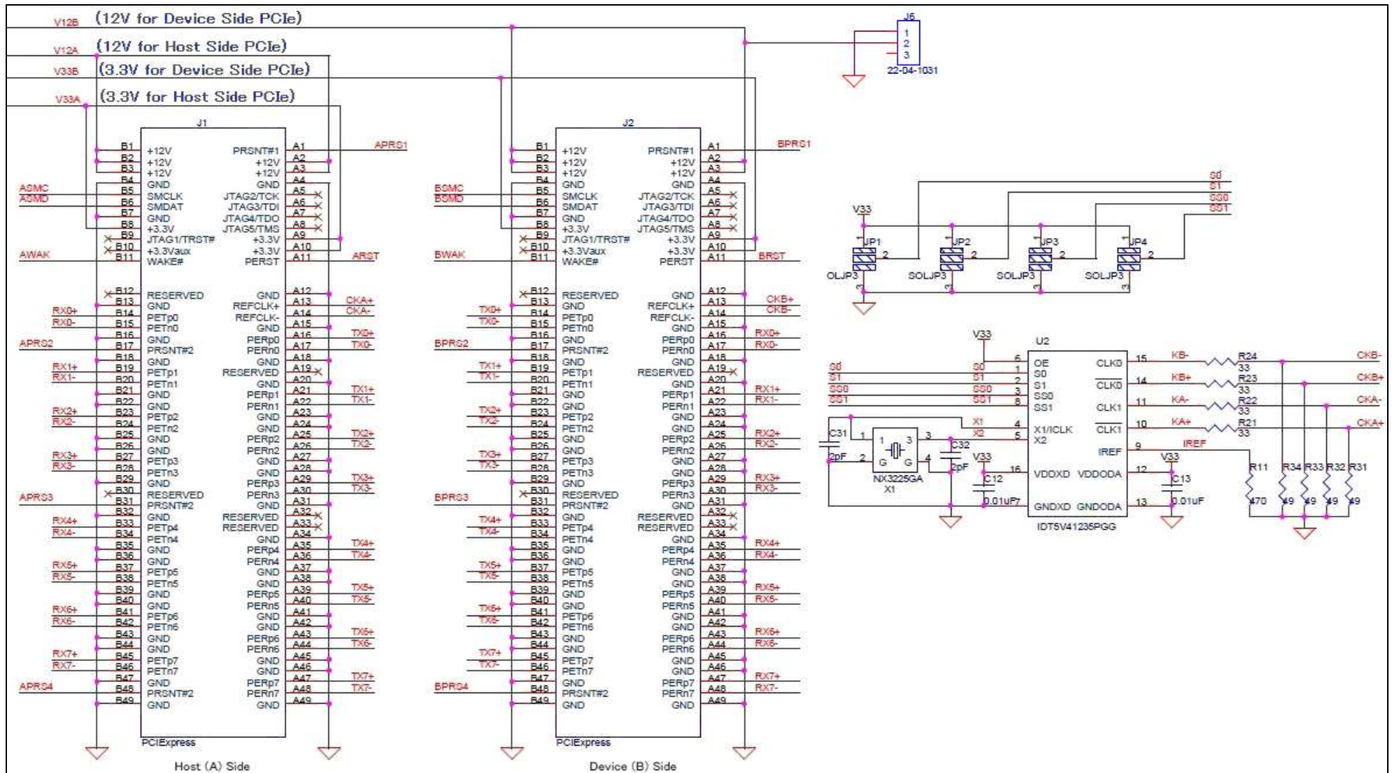
図 12: アダプタ回路図 (2/2)
