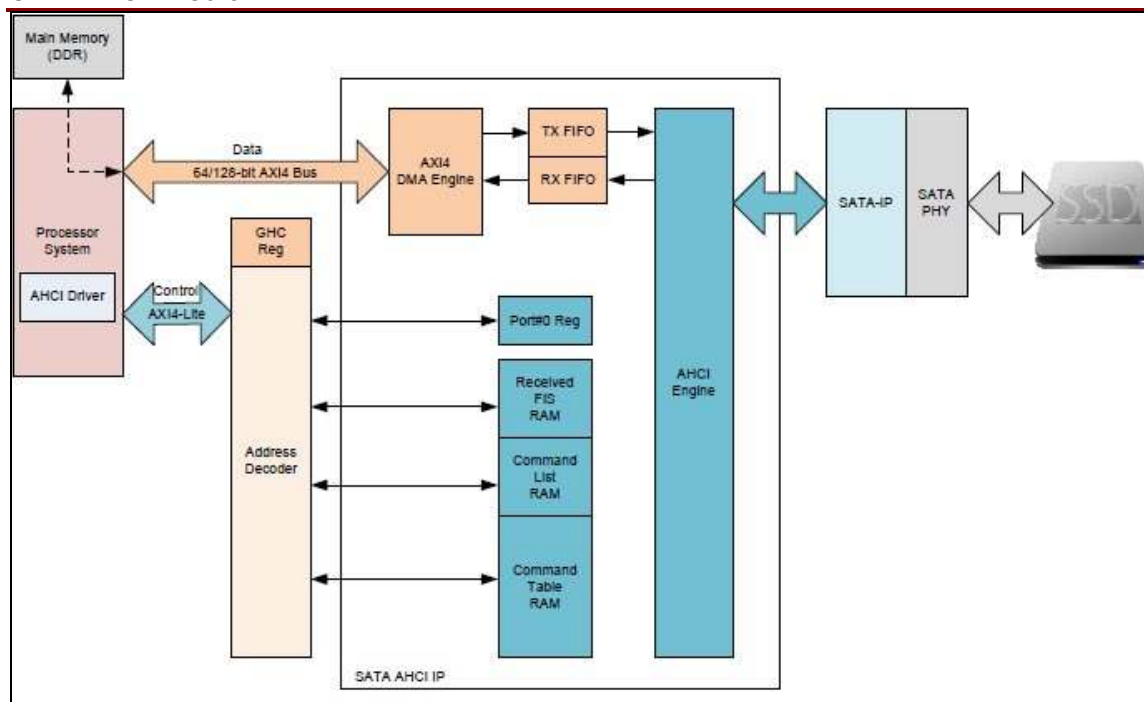
図1 : AHCI IP ブロック図
