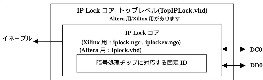
図 3 IP Lock コア トップレベル
