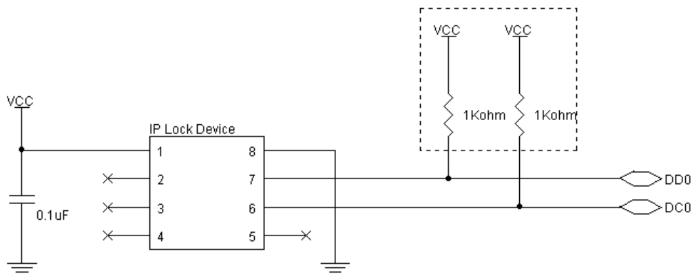
図 7 暗号処理チップ回路例
