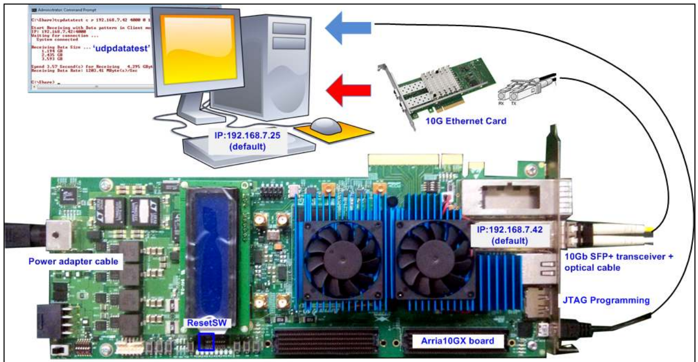
図 1-1: Arria10 GX ボードでの UDP10G-IP デモ環境
